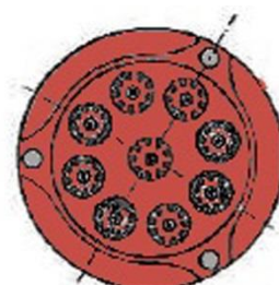
9 Innendüsen: F 28 A/D-9
