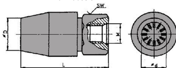
Wärmdüse STAR F-PM
