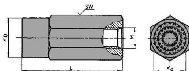
Wärmdüse Typ F-PMYE Gr. 12
